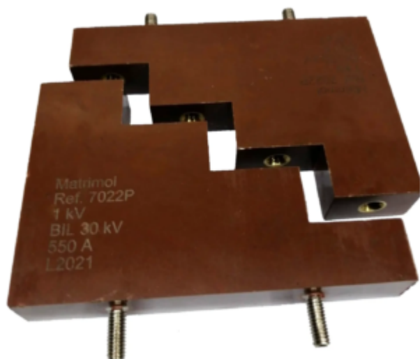
Aislador Resina Poliéster Bloque Distribución 550A
