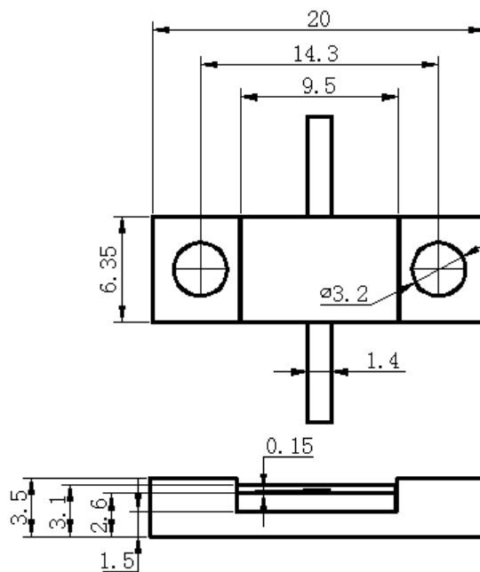
尺寸單位: mm
